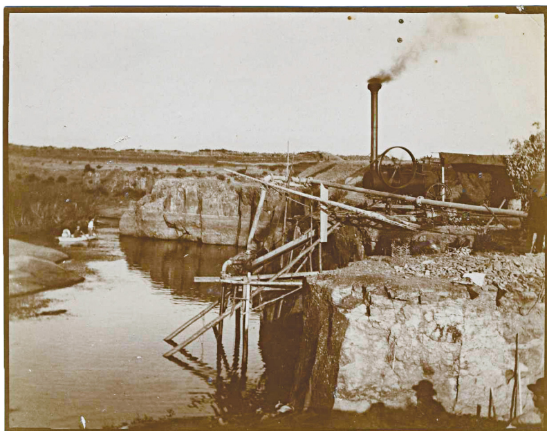
Fig. 10 – Pompaggio meccanico dell'acqua da una zona di cava al Palombaro, foto datata agosto 1909
