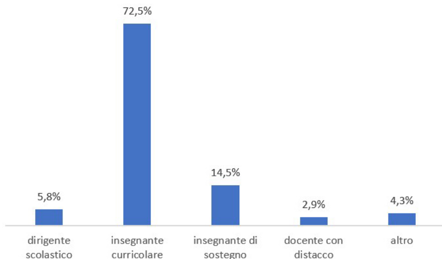
Figura 2. Ruolo partecipanti
